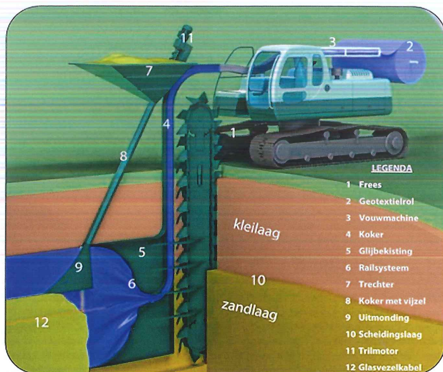
Deze schets laat zien hoe Piping Control werkt.
